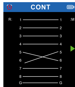
Пересечение пары
